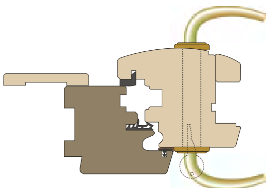
Particolare dell'ingombro serratura passante.
