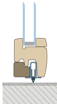
SOGLIA PARAFREDDO (le finestre con questa soluzione non sono garantite alla tenuta)
