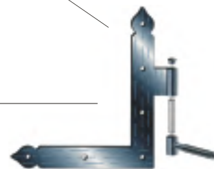
art: SQUADRO completo di CARDINE Per persiane, persiane balconi, sportelloni, sportelloni balcone, prime ante dx/sx
